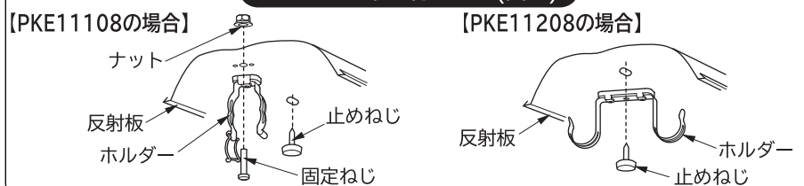
ホルダーの取り付けかた(図5)
