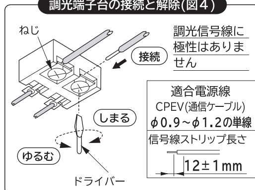
調光端子台の接続と解除(図4)
