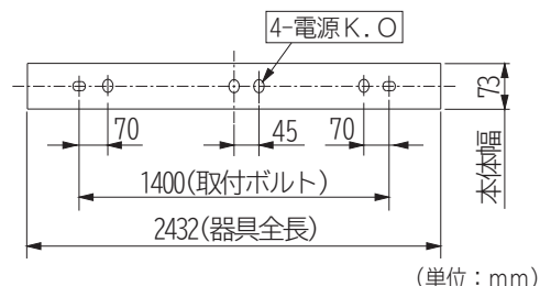
背面取付穴 (図1)
