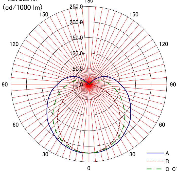
配光曲線
