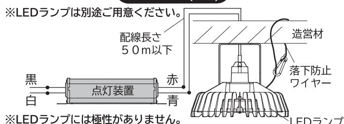
取付施工例(図4)
