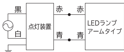
取付施工例(図4)
