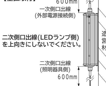
取付方向(図1)
