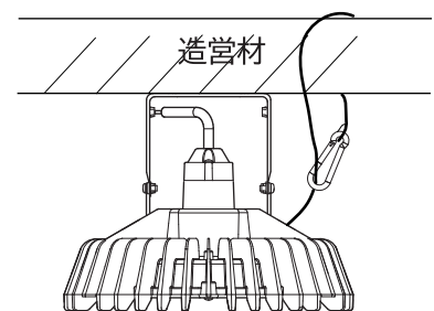
図3 落下防止ワイヤーの取り付け
