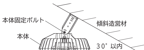
図5 傾斜造営材に取り付ける場合
