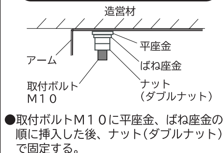
図2 LEDランプの取り付け
