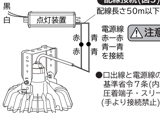
配線接続(図5)
