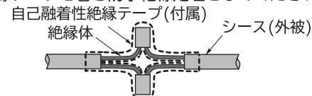
防水絶縁処理(図7)
