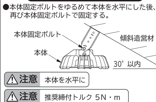
傾斜造営材に取り付ける場合(図6)
