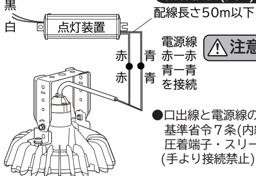
配線接続(図5)
