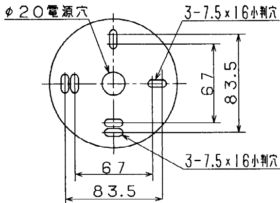
取付寸法図
