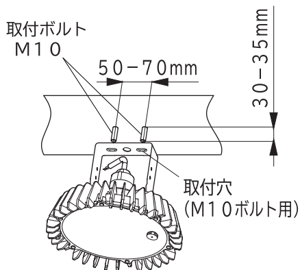
図2 取付ボルト施工寸法
