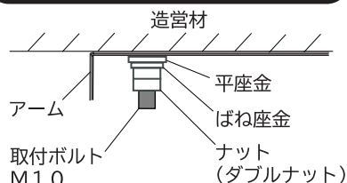
図3 LEDランプの取り付け
