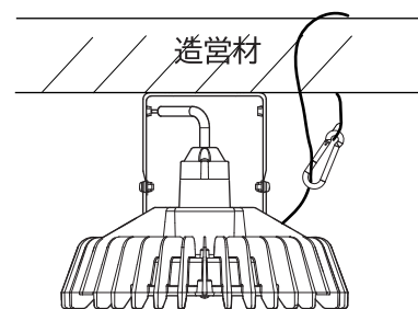
図4 落下防止ワイヤーの取り付け
