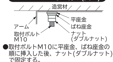
LEDランプの取り付け(図3)
