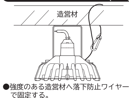
落下防止ワイヤーの取り付け(図4)
