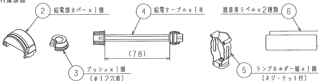
付属部品
