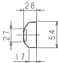
点灯装置断面寸法図
