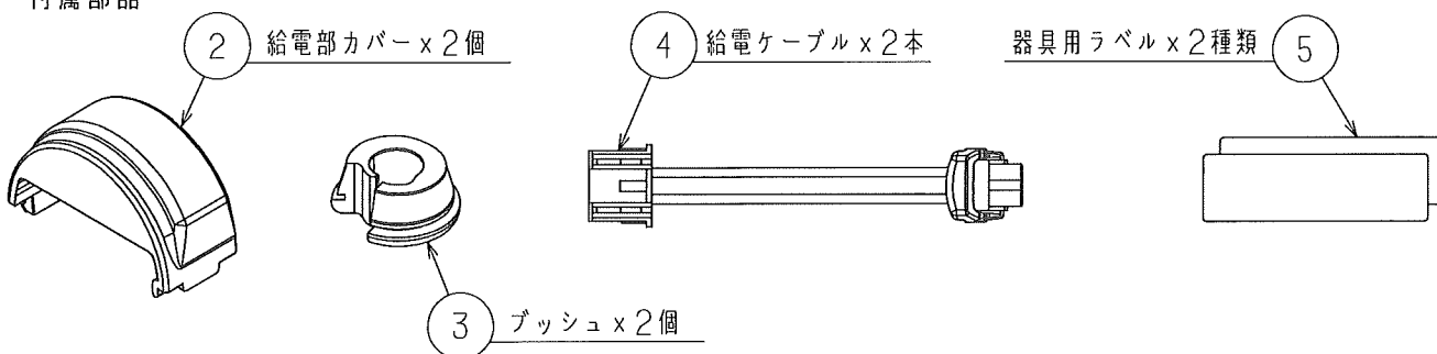
付属部品
