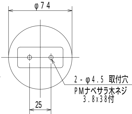
引掛シ - リング取付寸法図
