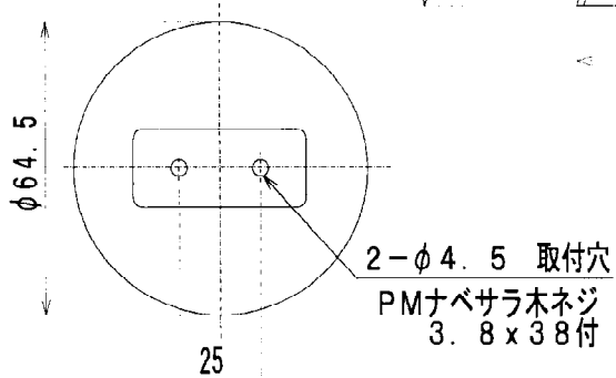
引掛シーリング取付寸法図
