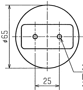
引掛シーリング取付寸法図
