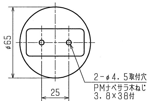
引掛シーリング取付寸法図
