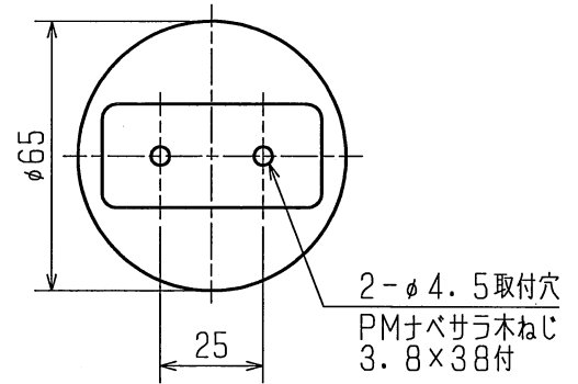
引掛シーリング取付寸法図
