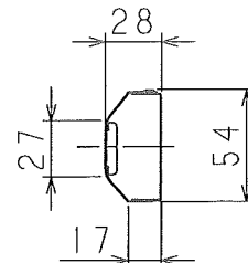
点灯装置断面寸法図
