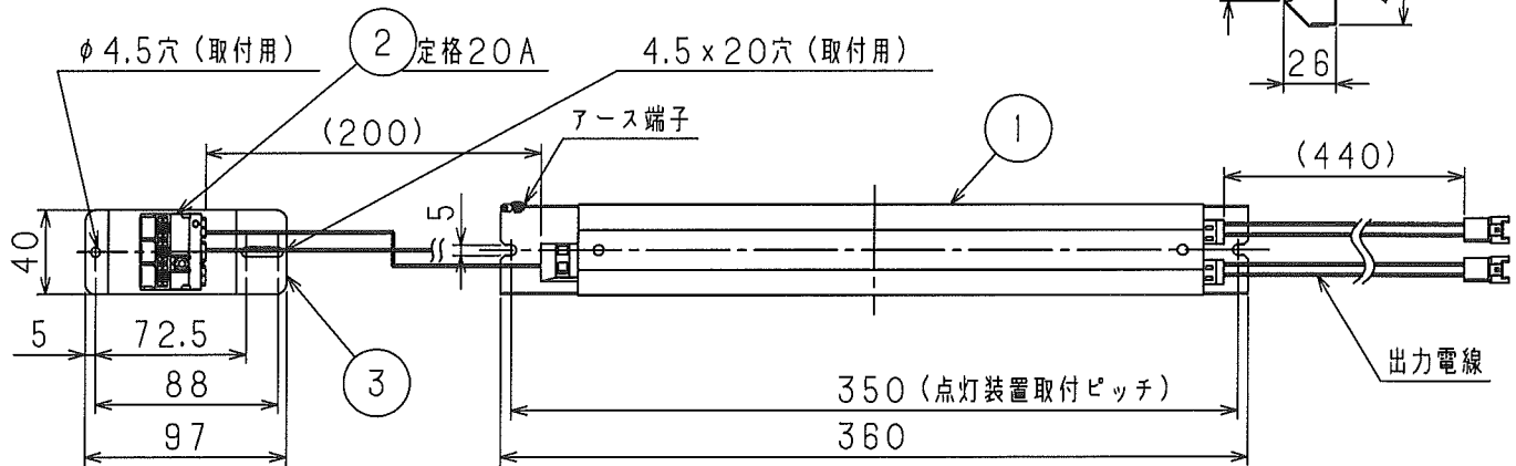
付属部品
