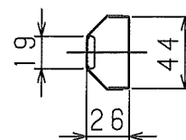
点灯装置断面寸法図
