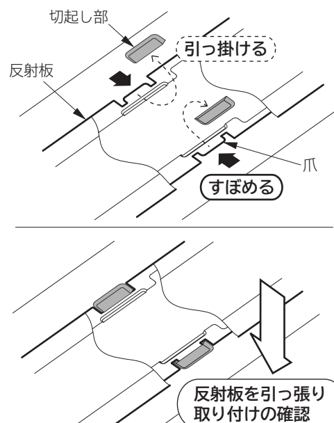
反射板の取り付けかた (図4)
