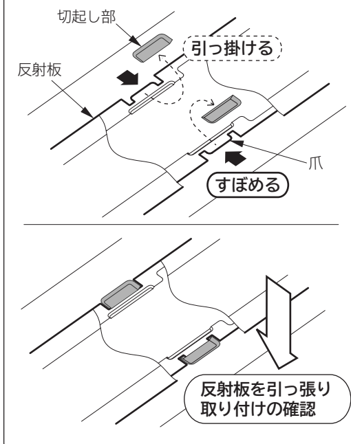
反射板の取り付けかた (図4)
