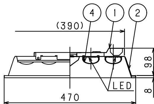
A 矢視
