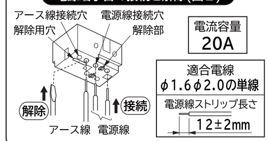
調光端子台の接続と解除(図3)
