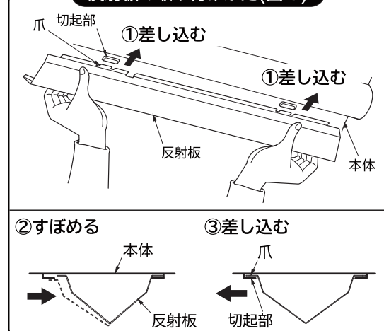
反射板の取り付けかた(図4)
