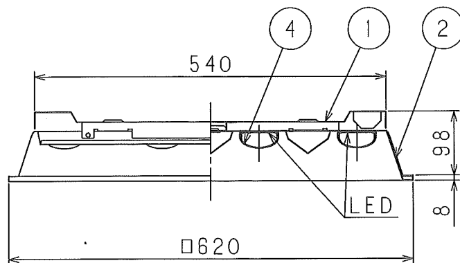
A 矢視
