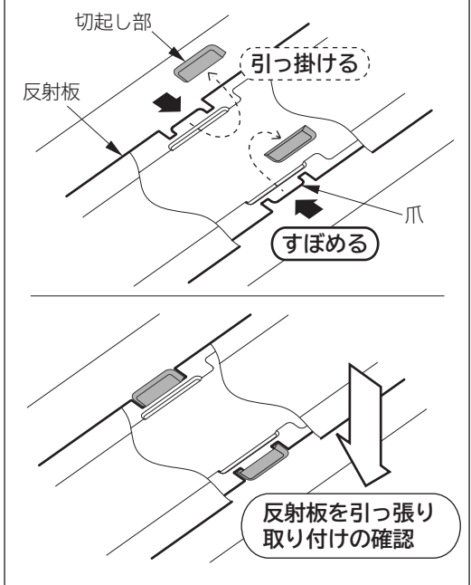
反射板の取り付けかた (図4)
