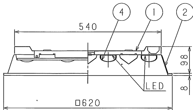
A 矢視
