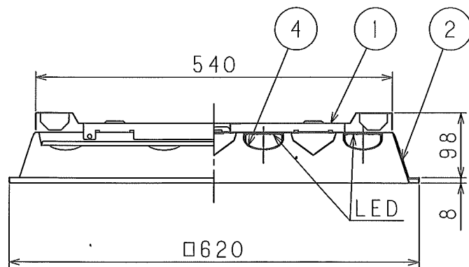
A 矢視
