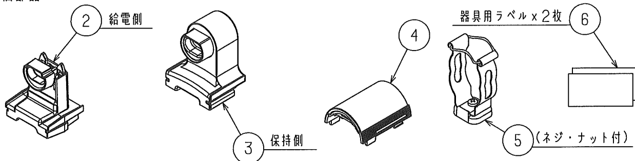
同梱部品
