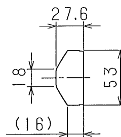
点灯装置断面寸法図
