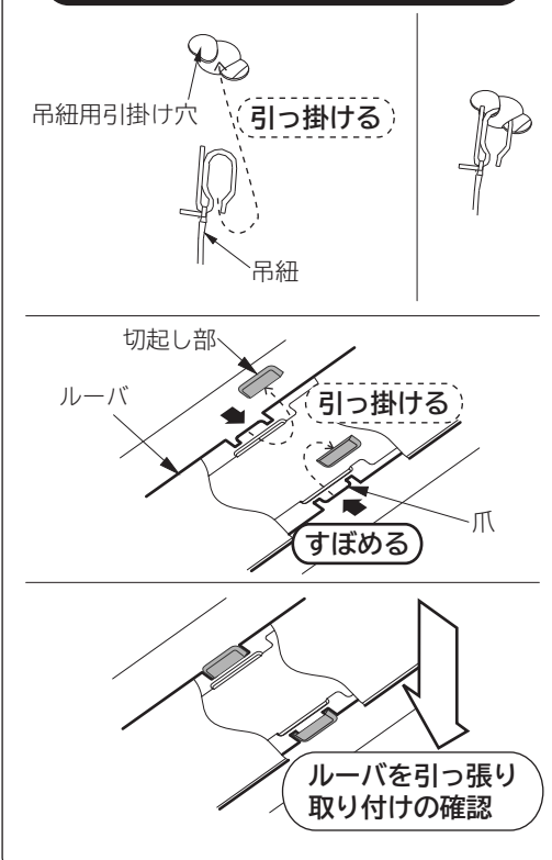
ルーバの取り付けかた (図4)
