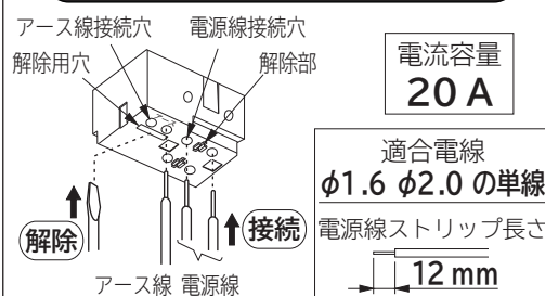
調光端子台の接続と解除 (図3)
