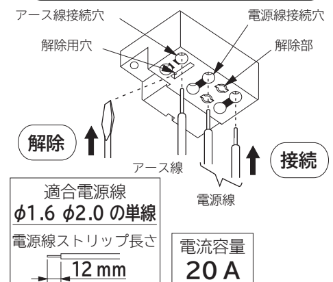
電源端子台の接続と解除 (図4)
