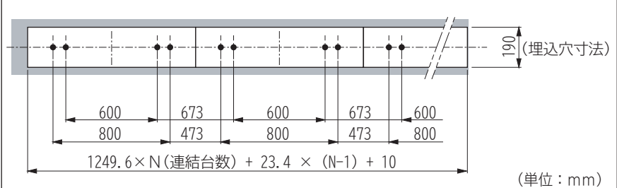
連結のしかた (図3)
