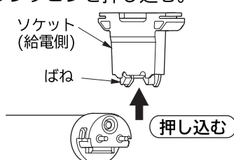
直管形LEDランプの取り付けかた(図5)
