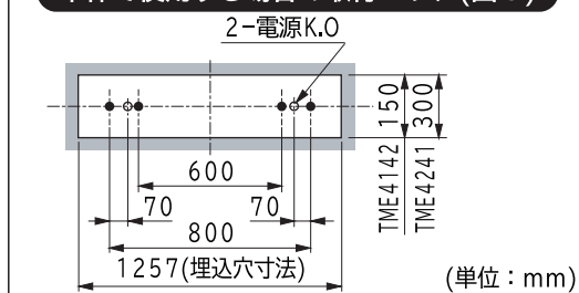
単体で使用する場合の取付ピッチ(図1)
