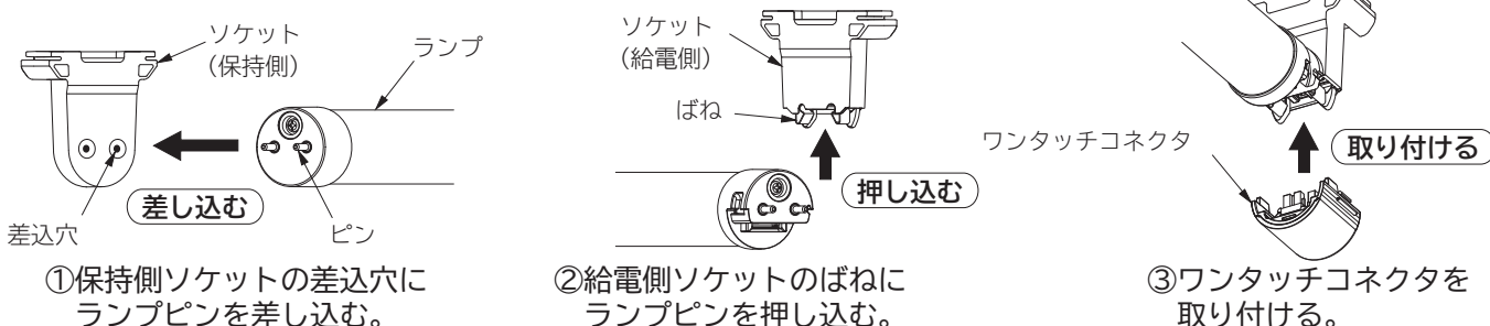
ランプの取り付けかた (図5)
