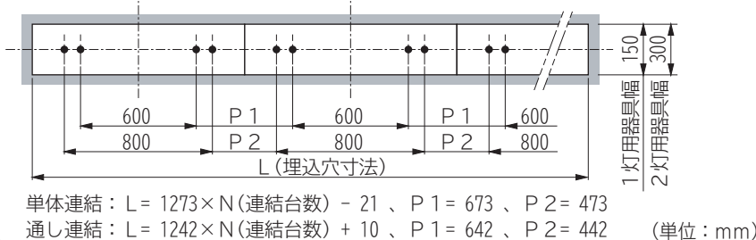
本体と反射板の連結 (図3)
