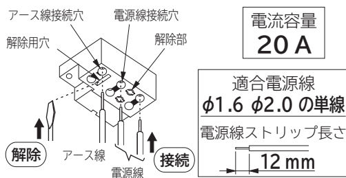
電源端子台の接続と解除 (図4)
