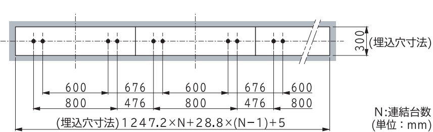
連結のしかた(図3)
