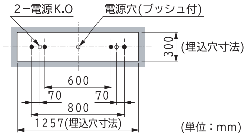
単体で使用する場合の取付ピッチ(図1)
