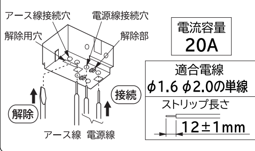
電源端子台の接続と解除(図4)
