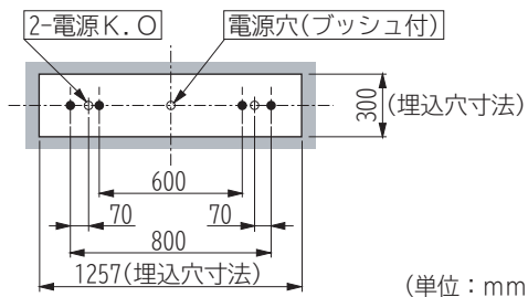
単体で使用する場合の取付ピッチ（図1）
