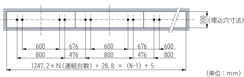
単体N台連結で使用する場合の取付ピッチ（図2）
