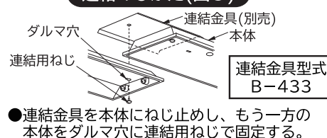
電源端子台の接続と解除(図4)
