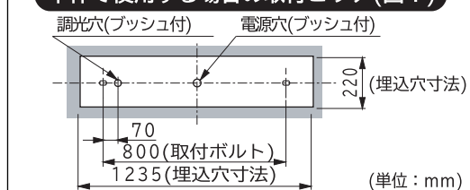
単体で使用する場合の取付ピッチ(図1)
