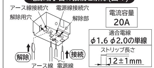
調光端子台の接続と解除(図5)
