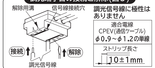
調光端子台の接続と解除(図5)
