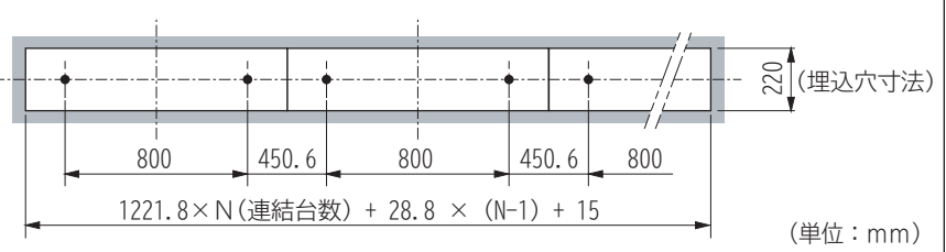
単体N台連結で使用する場合の取付ピッチ(図2)
