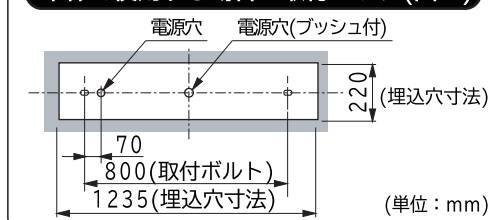
単体で使用する場合の取付ピッチ(図1)
