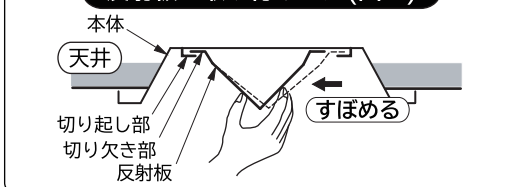
反射板の取り付けかた(図5)
