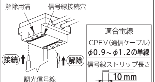
反射板の取り付けかた (図4)
