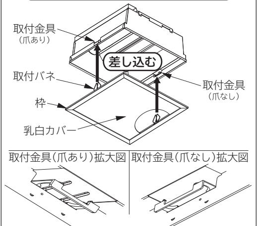
乳白カバーの取り付けかた (図5)
