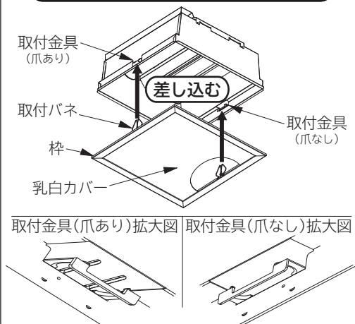
乳白カバーの取り付けかた (図5)
