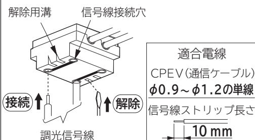
反射板の取り付けかた (図4)
