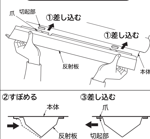
反射板の取り付けかた(図4)
