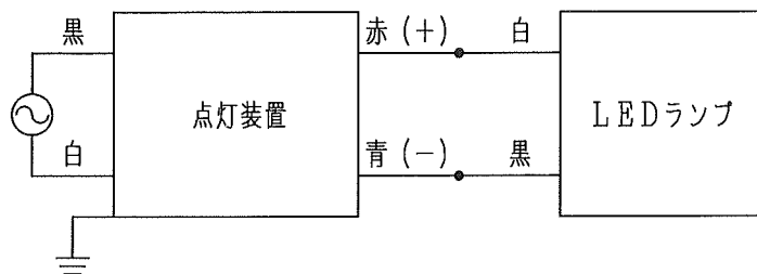
〔結線図〕
