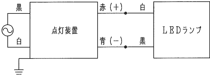
〔結線図〕
