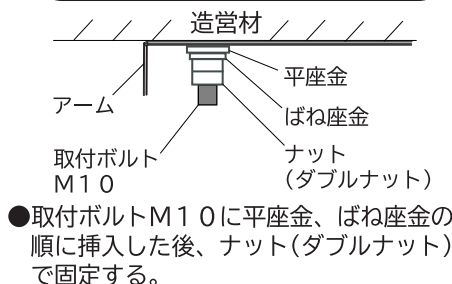
図2 LEDランプの取り付け
