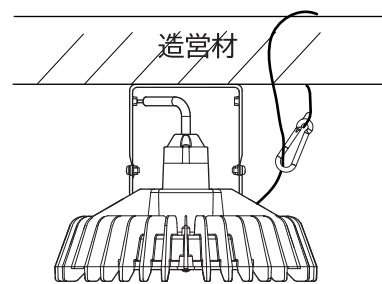
図3 落下防止ワイヤーの取り付け
