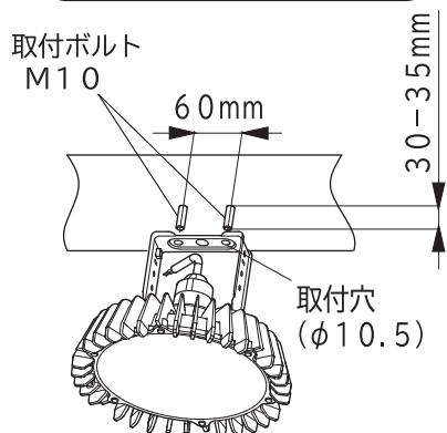
図1 取付ボルト施工寸法
