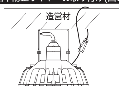
落下防止ワイヤーの取り付け(図3)
