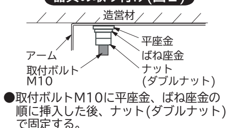
器具の取り付け(図2)
