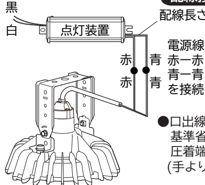
配線接続(図4)
