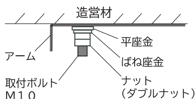
図2 LEDランプの取り付け
