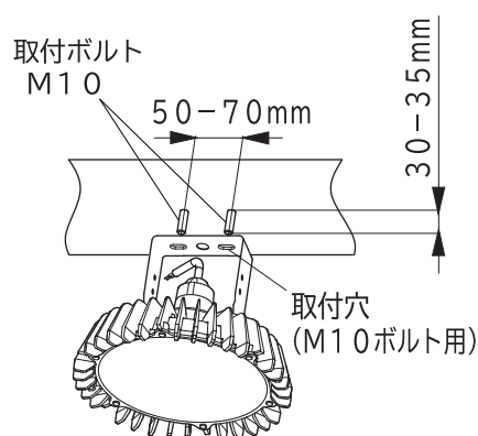
図1 取付ボルト施工寸法
