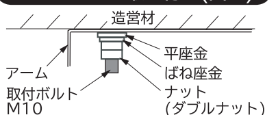
LEDランプの取り付け(図2)
