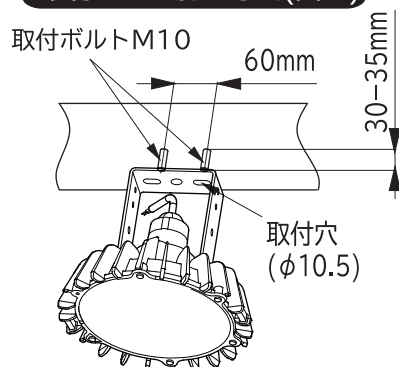
取付ボルト施工寸法(図1)
