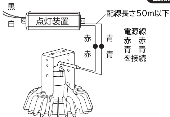
配線接続(図4)
