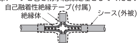
防水絶縁処理(図5)
