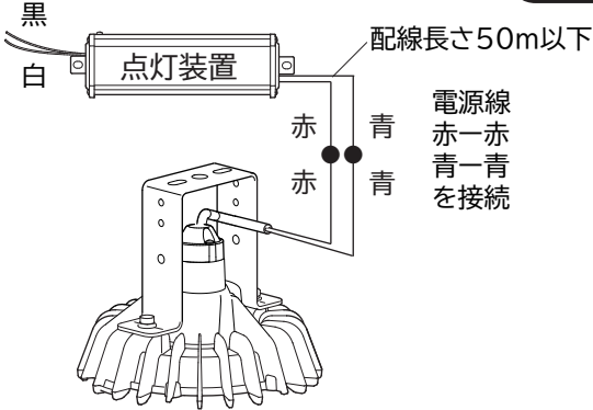
配線接続(図4)
