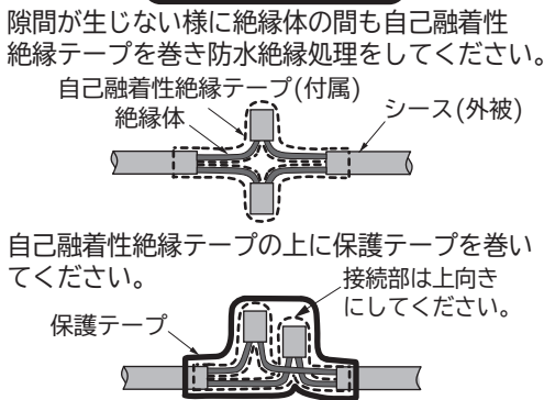
防水絶縁処理(図5)
