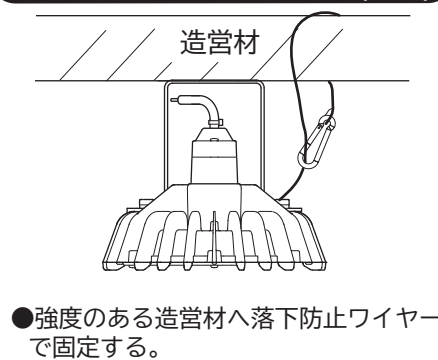
落下防止ワイヤーの取り付け(図3)
